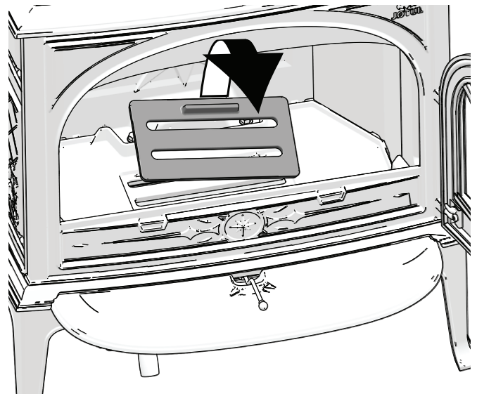
Rys. 20 Wymiana rusztu
