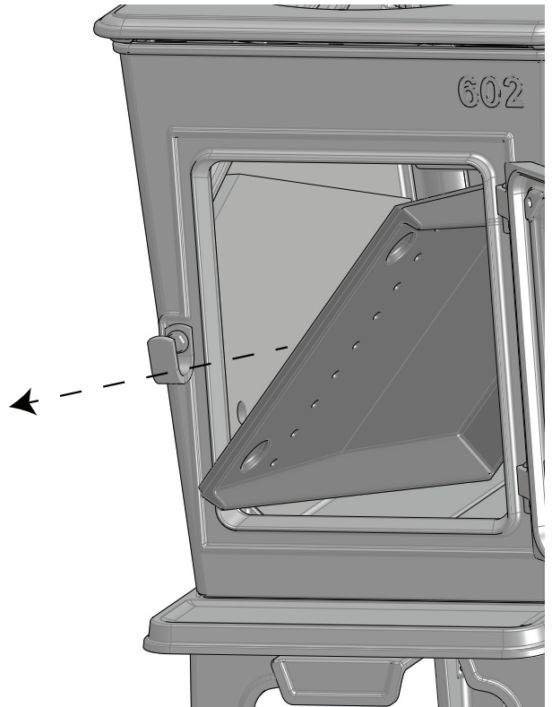
Fig. 23 Fjernelse af røgvenderplade
