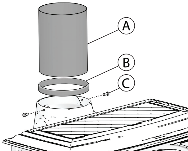
Afb. 6 Monteren van kachelpijp
