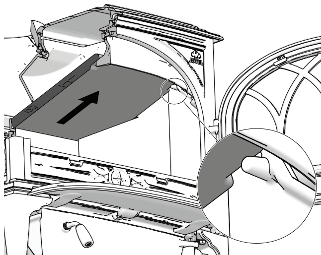
Fig. 16a Lossa rökhylja
