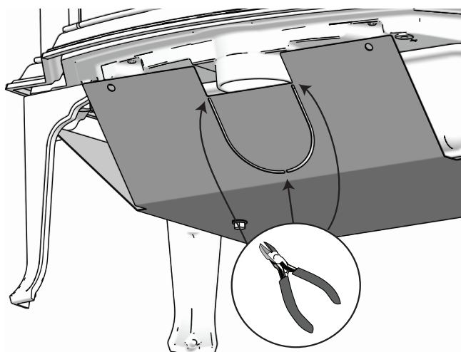
Fig. 8a Montering av frislutstillförsel
