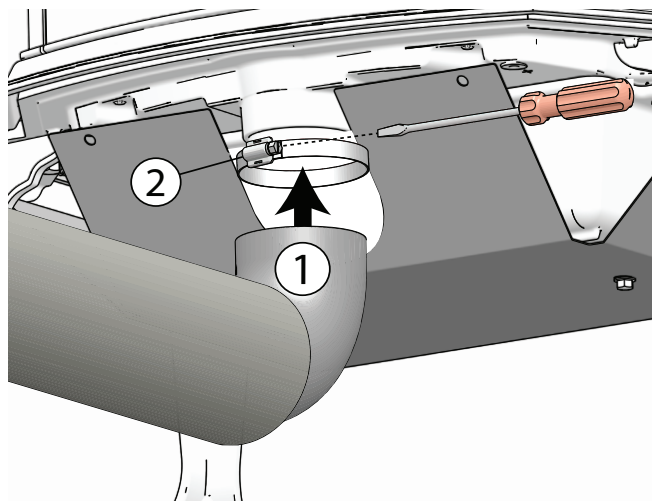
Fig. 8b Montering av frislutstillförsel
