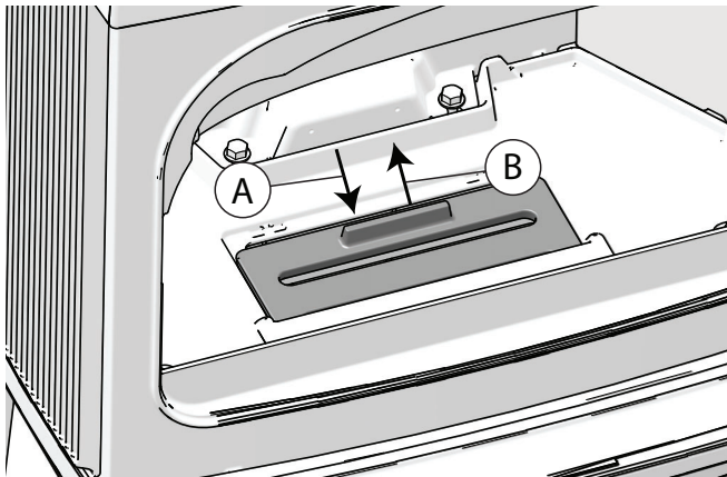
Kuva. 13 Tuhkaritilä
