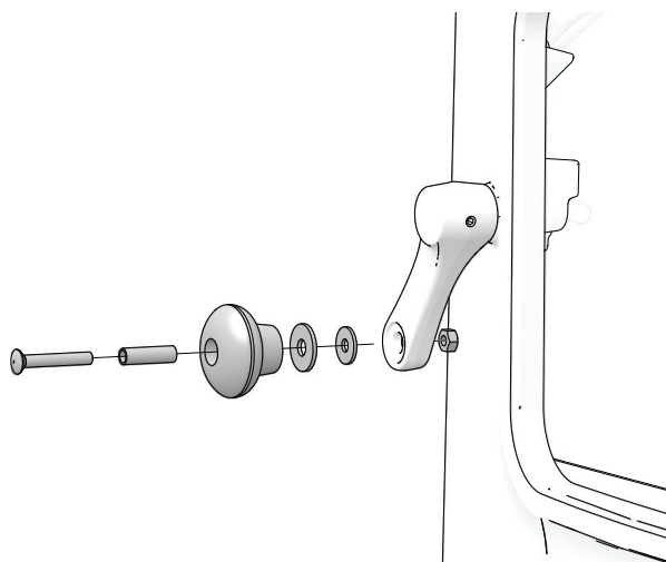
Fig. 3 Handtag montering
