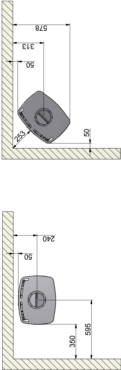
Mindestabstände zu brennbaren Materialien (ohne Seitenfenster)
