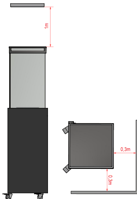
Fig 2 – Minimumsavstander
