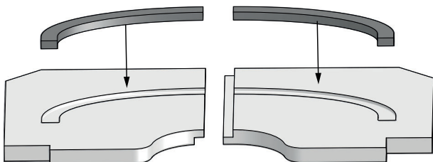
Abb. 18c Austausch der Dichtung auf dem Leitblech
