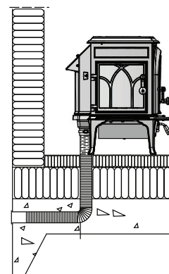
Abb.9b Durch Fußboden und Bodenplatte
