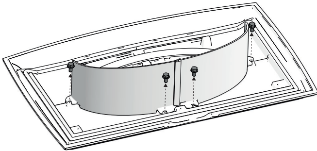
Afb. 19d Vervangen van uitlaatplaat
