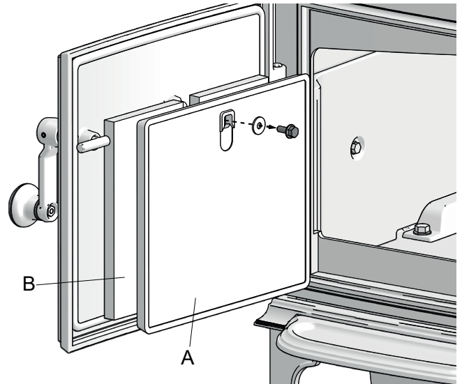
Afb. 23 Vervangen branderplaat op zijdeur
