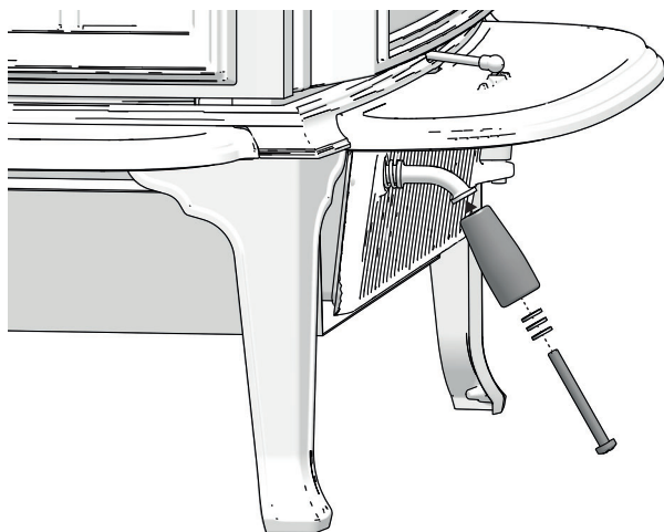
Afb. 4b Monteren van hendel deur aslade
