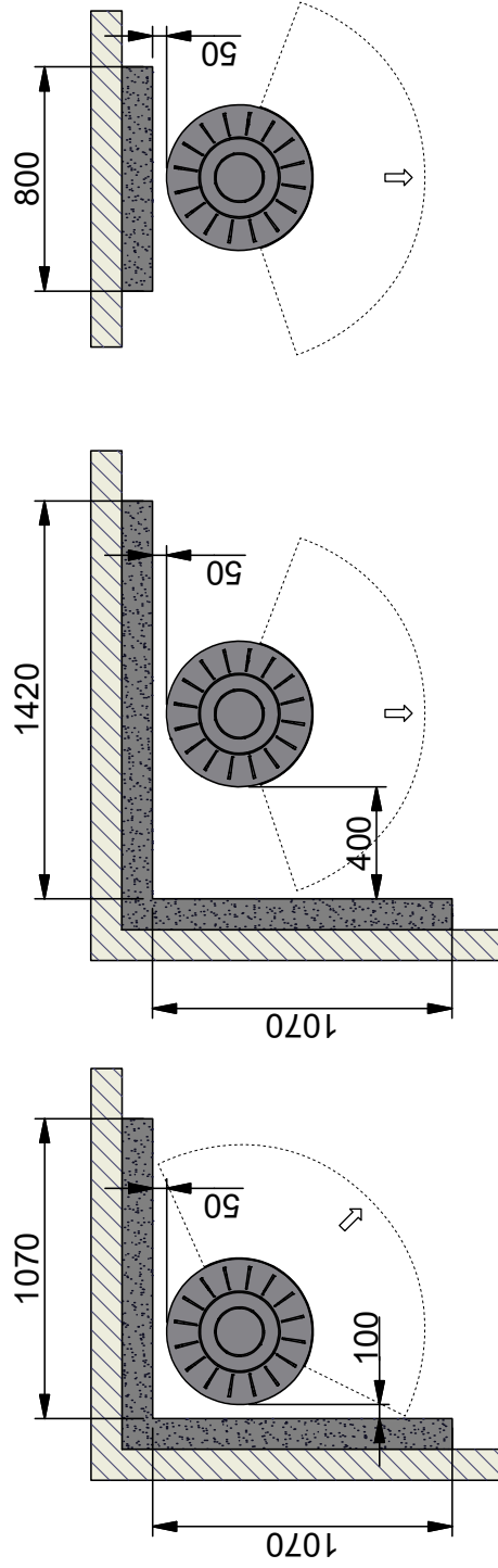
Mindestabstände zur brennbaren Wand, geschützt mit Brandschutzwand
