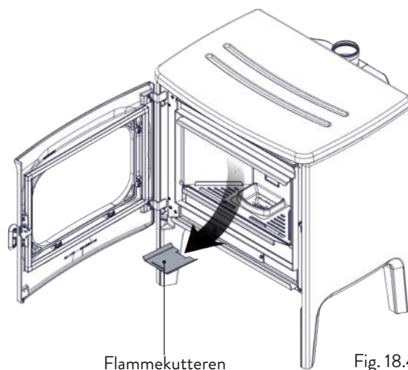
Forbrenningskammer
