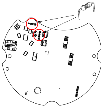
Figure 27 : Convertisseur à 1 connecteur
