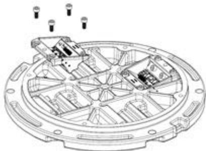
Figure 17 : Retirez le support de la carte à LED
