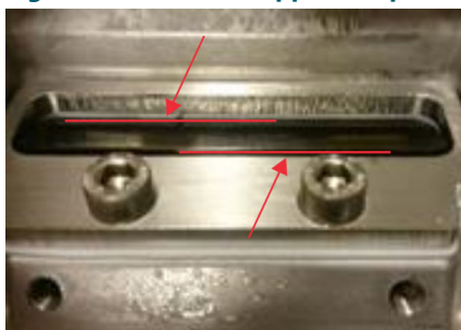
Figure 20 : Bord du support de prisme
