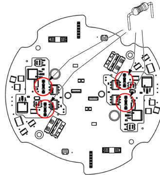
Figure 28 : Convertisseur à 2 connecteurs
