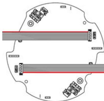
Figure 11 : Convertisseur à 2 connecteurs
