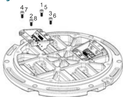
Figure 15 : Serrez les vis
