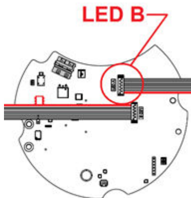
Figure 10 : Convertisseur à 1 connecteur
