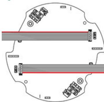
Figure 23 : Convertisseur à 2 connecteurs
