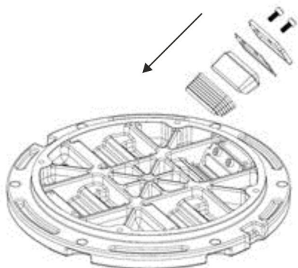
Figure 19 : Nouveau joint de prisme dans le prisme
