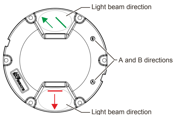
Figure 5 : Directions d'émission de la lumière
