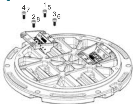
Figure 21 : Serrez les vis dans l'ordre
