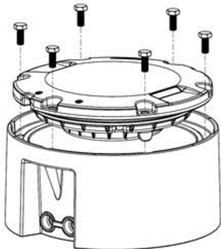
Figure 3 : Feux à base peu profonde de 12 pouces, classe 1, à montage direct
