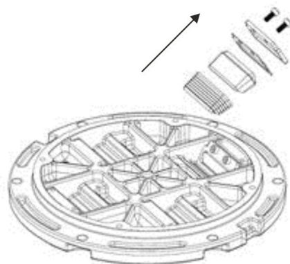
Figure 18 : Retirez le prisme et le joint
