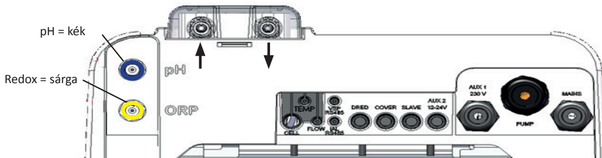
A vezérlőegység alulnézete telepített modulal
