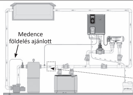
Telepítés fűtőrendszerrel
