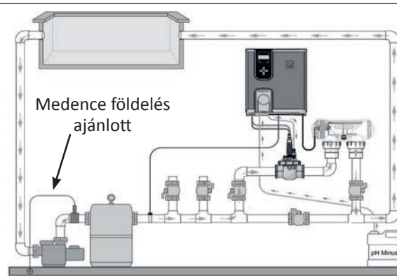
By-pass telepítés
