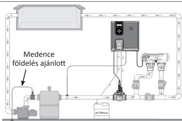
Soros telepítés
