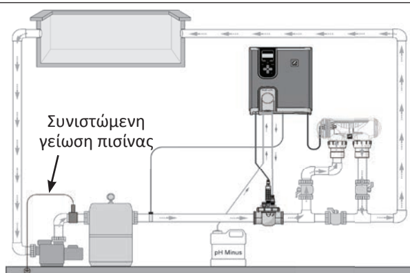
Εγκατάσταση σε σειρά
