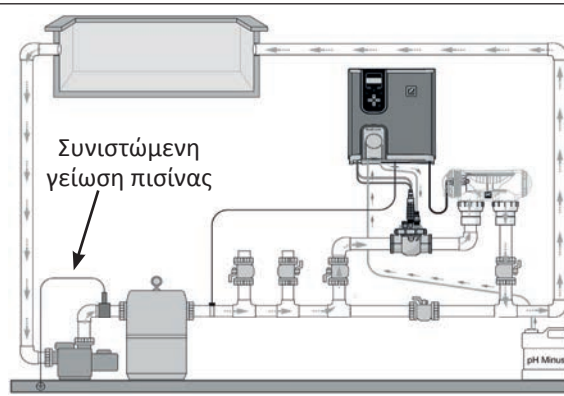
Εγκατάσταση με παράκαμψη
