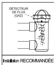
Installation RECOMMANDÉE
