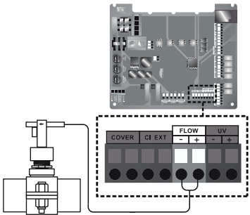
Ligação do sensor de palhetas (fluxostato) à placa principal.
