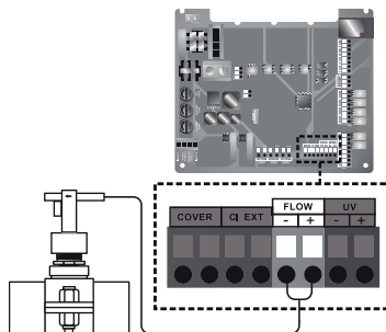
Connexion de la sonde inter Débit (flussostat) à la carte principale.
