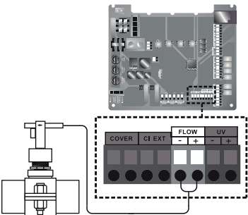
Aansluiting van de switchsensor (stromingssensor) op het moederbord.
