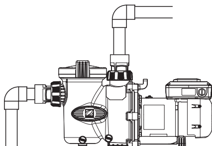
FIGURA 2 - INSTALAÇÃO CORRETA
