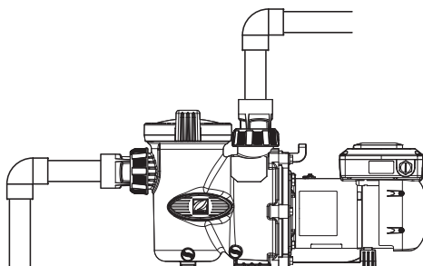
FIGURA 2 - INSTALLAZIONE CORRETTA
