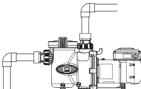
FIGURA 2 - INSTALAÇÃO CORRETA
