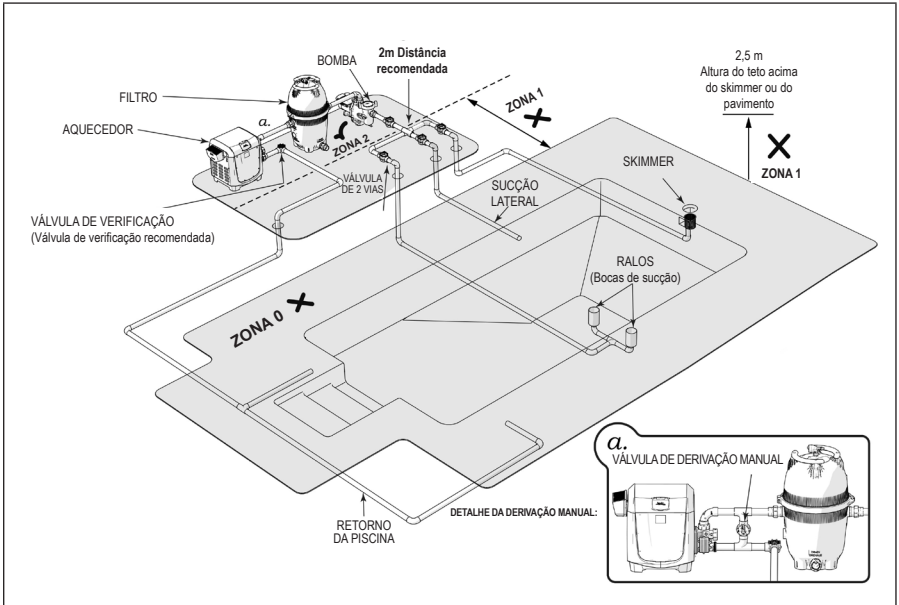
FIGURA 1 - INSTALAÇÃO DA TUBAGEM PADRÃO
