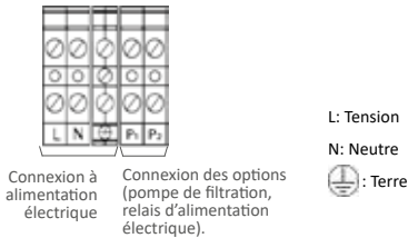
Bornier pour alimentation monophasée
