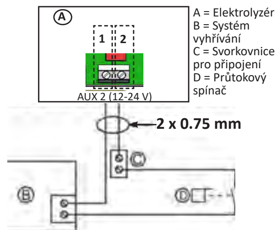
Zapojení systému vyhřívání bez dálkového řízení zapnutí/vypnutí
