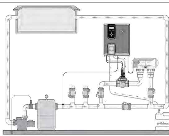
Instalace elektrolyzáru + volitelného modulu
