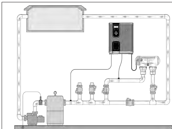
Instalace vlastního elektrolyzáru
