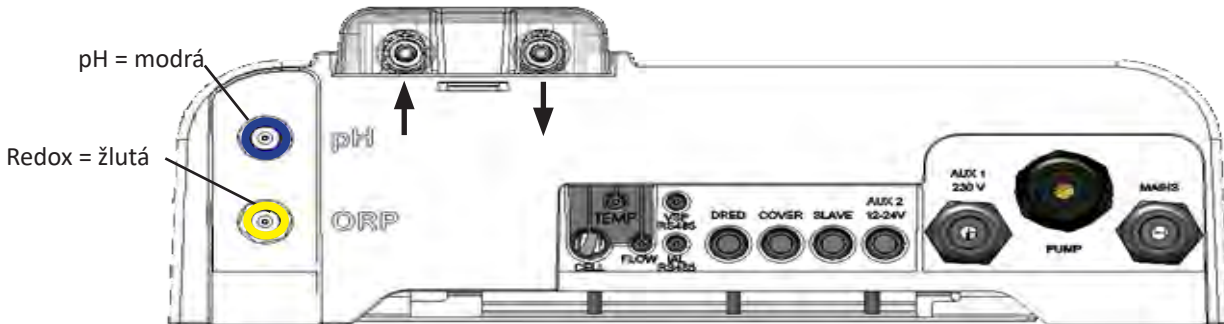
Pohled zespodu na ovládací skřín s instalovaným modulem
