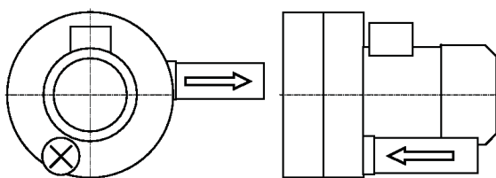
Fig. 3: Turbinas de canal lateral de doble etapa (dos rodetes en serie) Double stage side channel blower (2 impellers in serial) Soufflante bi-étagée à canal latéral (2 roues à aubes en série) Series: HSCxxxx-2S...
