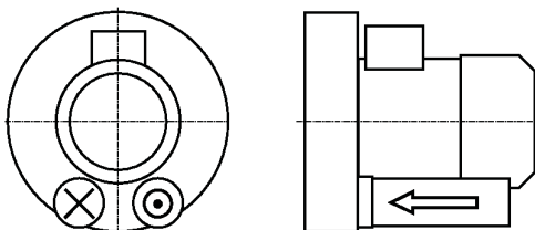
Fig. 1: Turbinas de canal lateral de simple etapa (1 rodete) Single stage side channel blower (1 impeller) Soufflante mono-étagée à canal latéral (1 roue à aubes) Series: HSCxxxx-1M...
