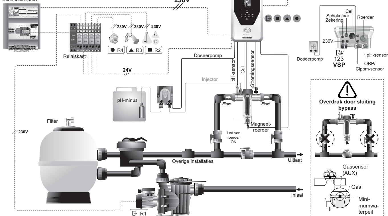
Schakelschema
