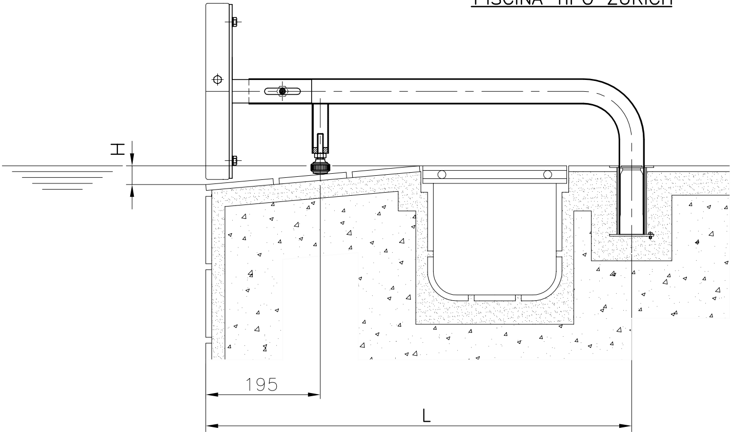
PISCINA TIPO FINLANDES
