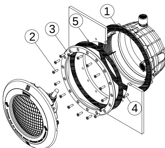
PREFABRICATED POOL PISCINA PREFABRICADA
