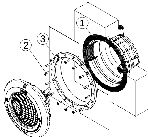
CONCRETE POOL WHIT LINER PISCINA DE HORMIGÓN CON LINER
