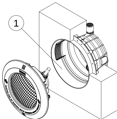
CONCRETE POOL PISCINA DE HORMIGÓN
