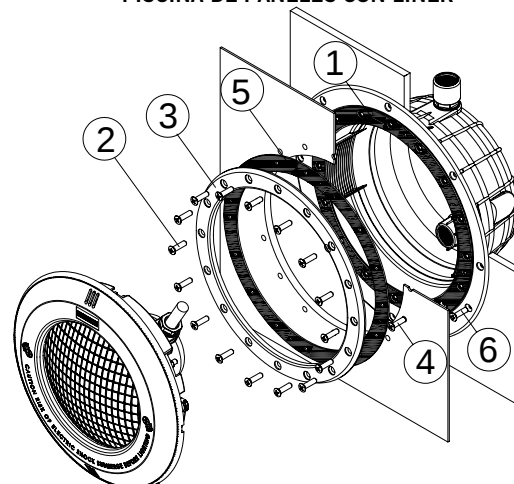
PANELLED POOL WHIT LINER PISCINA DE PANELES CON LINER
