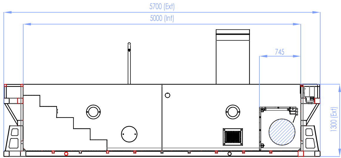
B-B
