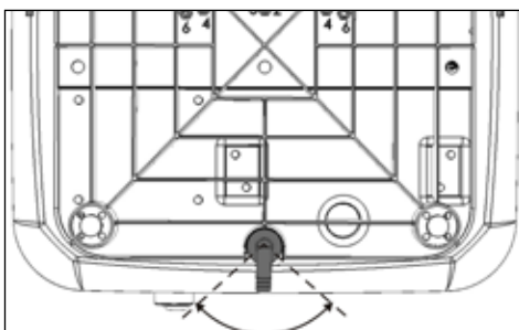
Orientação da evacuação dos condensados (vista de baixo do aparelho)
