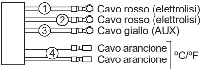
Collegamento del sensore di flusso di gas al dispositivo.
