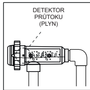
POVOLENÁ INSTALACE ALLE MODELLEN (Model 12/24/32 LS g/h s průtokovým senzorem)
