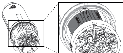
INSTALLAZIONE CONSENTITA TUTTI I MODELLI (Mod. 12/24/32 LS g/h con sensore di flusso)
