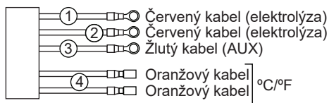
Připojení senzoru průtoku plynu k zařízení.
