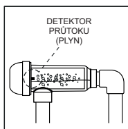
POVOLENÁ INSTALACE ALLE MODELLEN (12/24/32 g/h modely s průtokovým senzorem)
