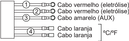
Ligação do sensor de fluxo de gás ao dispositivo.
