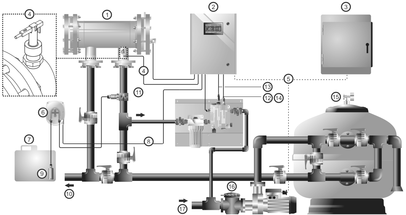
Fig.3 DIAGRAMA DE INSTALACIÓN UNA CELULA PARA VERSIONES CON EXTENSIÓN DE CONTROL EXT-1E O EXT-2 INTEGRADA.
