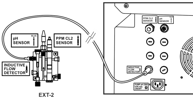
Fig. 10b , Ext-2 (Ver Fig 3)
