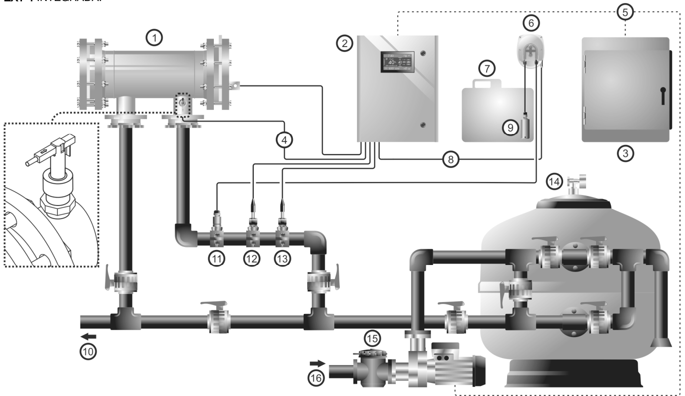
Fig.1 DIAGRAMA INSTALACIÓN UNA CELULA, MOD-50, 80,120,180,300 EX / EX(M) Y D-50,80,120 EX LS. TAMBIEN MODELOS CON EXT-1 INTEGRADA.
