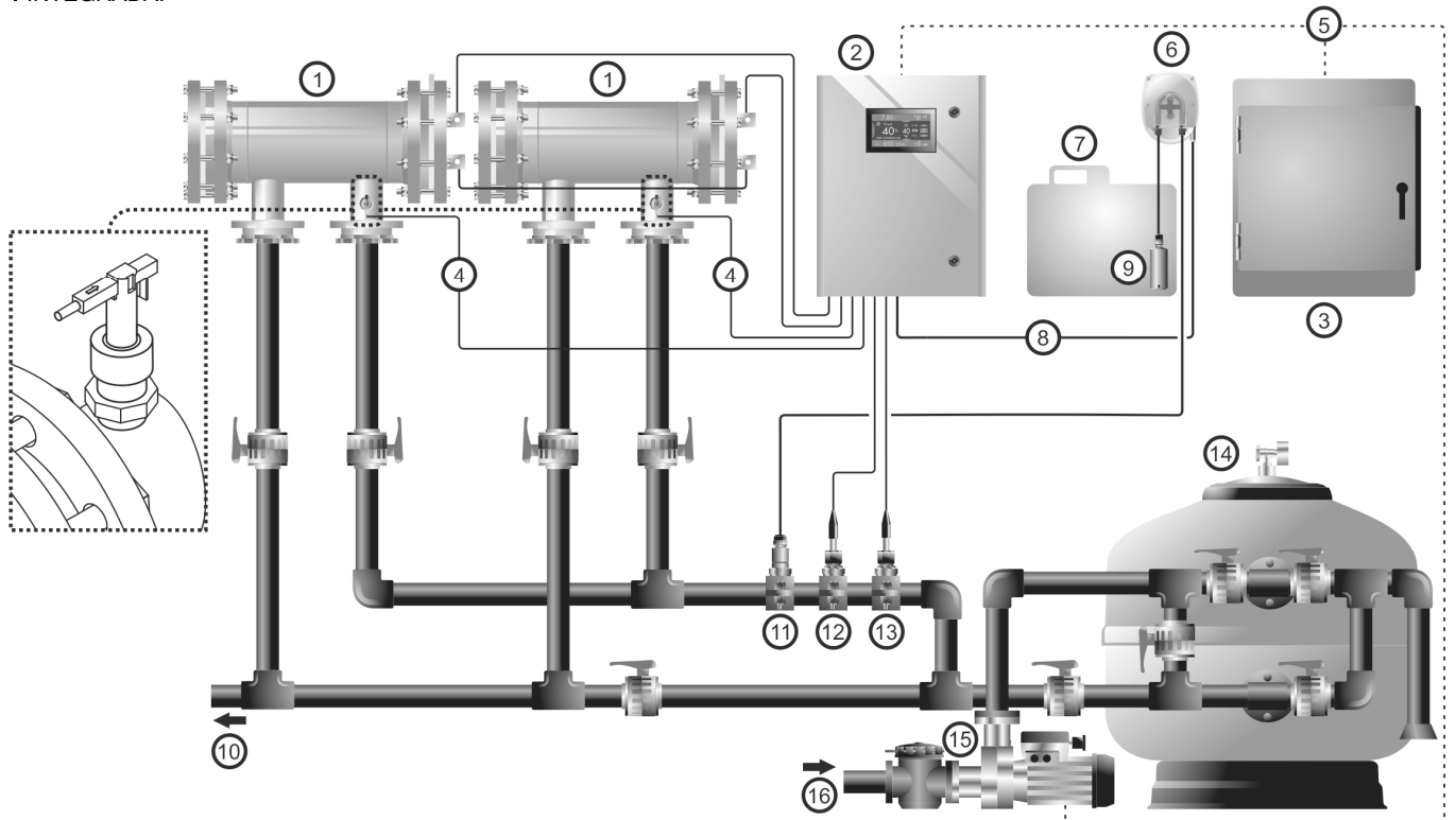
Fig.2 DIAGRAMA INSTALACIÓN DOS CELULAS, MOD-600 EX / EX(M), MOD-300 EX LS, MOD-180 EX LS; TAMBIEN MODELOS CON EXT-1 INTEGRADA.
