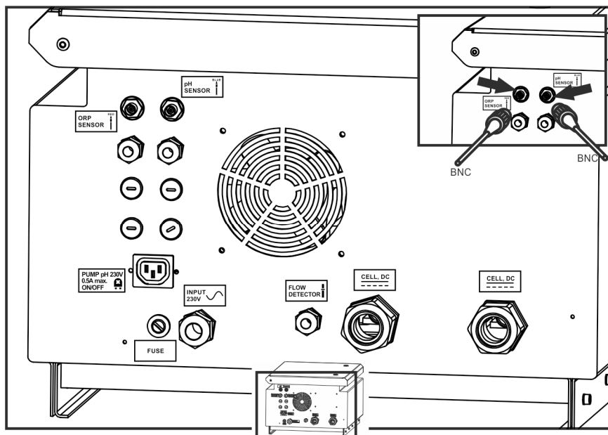
EJEMPLO CONEXIONADO EXT-1
