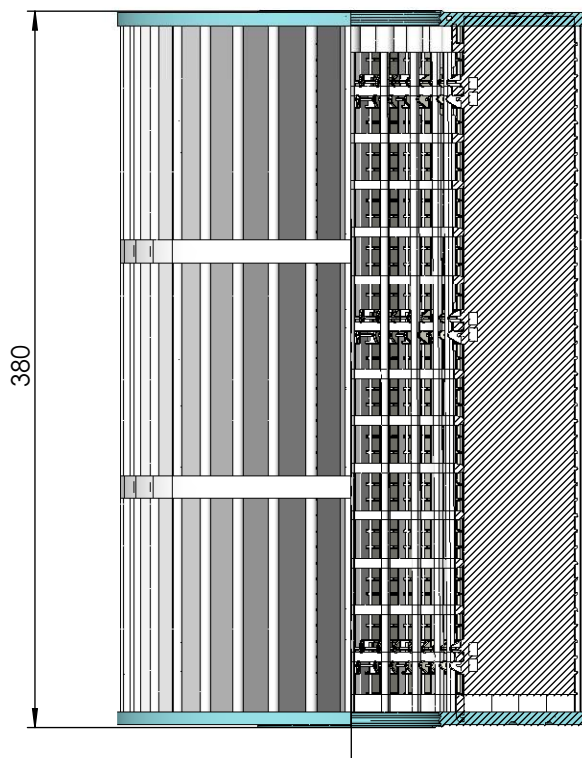
SECCIÓN A-A
