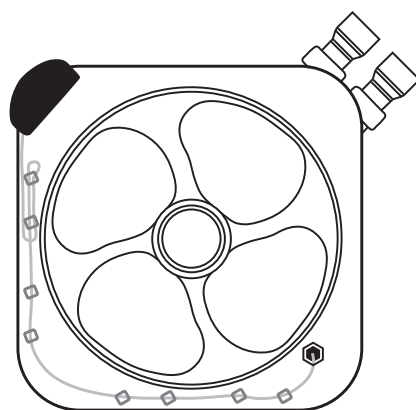
Kabelns dragning om användargränssnittet vrids åt vänster
