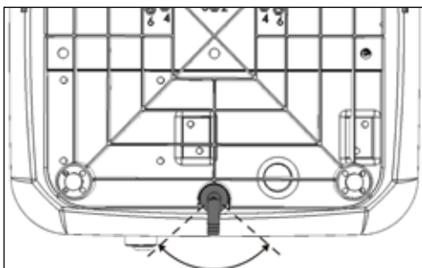
Ориентация на изтичането на кондензат (изглед от долната страна на уреда)
