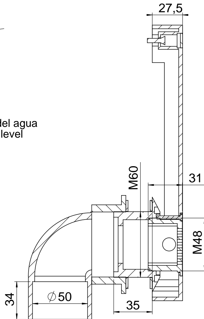
SECCIÓN A-A ESCALA 1 : 2
