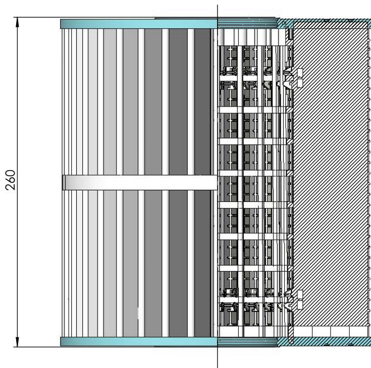
SECCIÓN A-A
