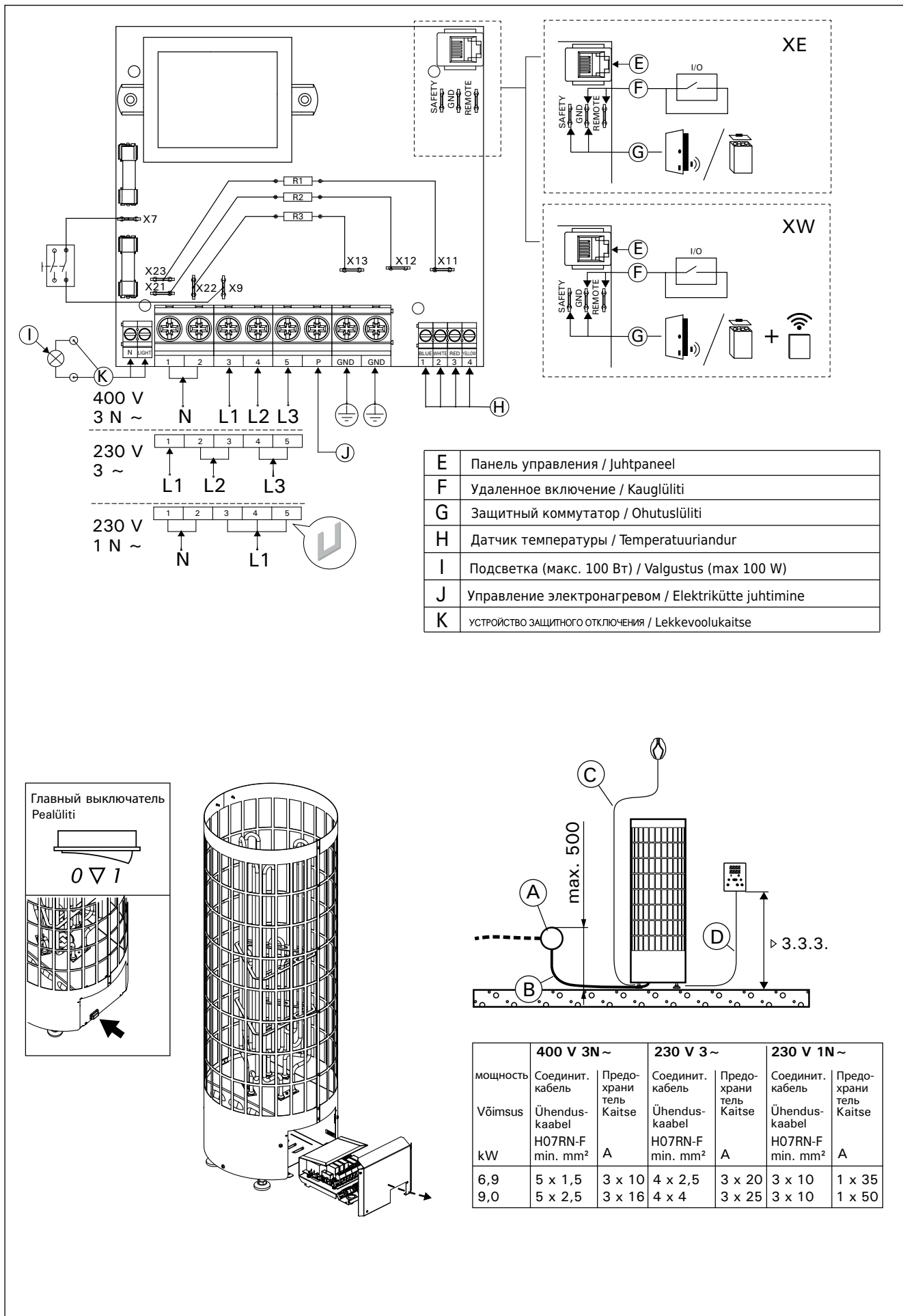
Рисунок 7. Электромонтаж Joonis 7. Elektriühendused
