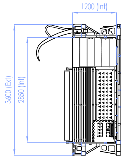
A-A
