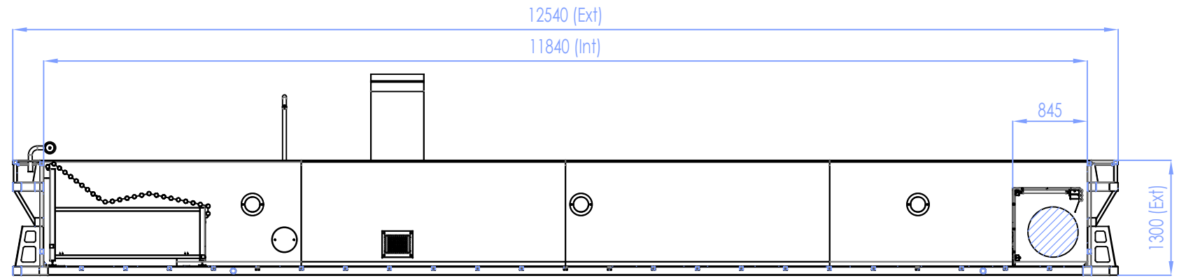
B-B
