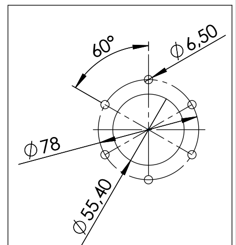
DIMENSIONES TROQUEL
