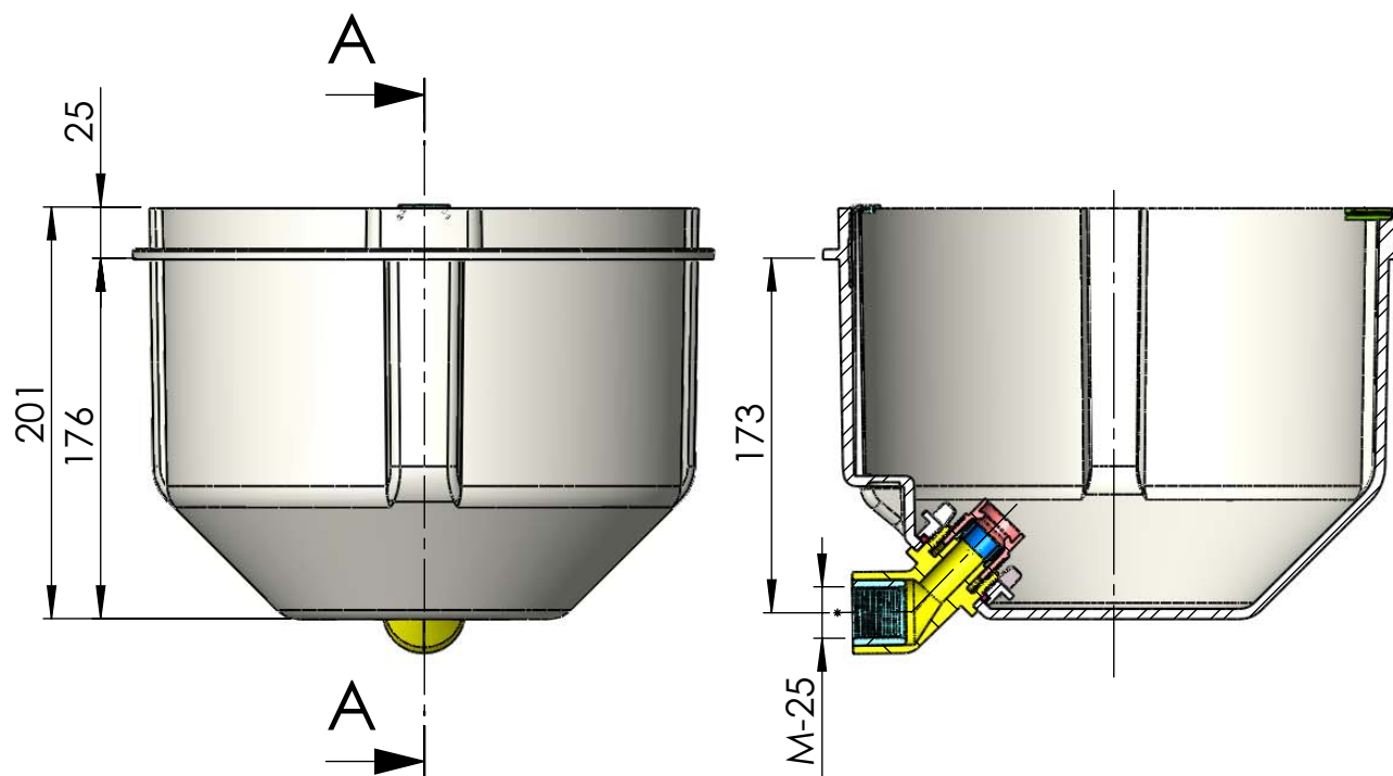
SECCIÓN A-A
