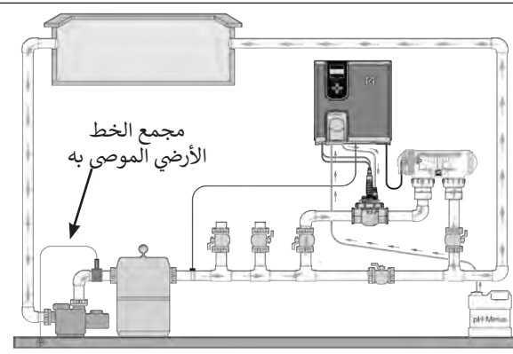
التركيب على صمام تحويل
