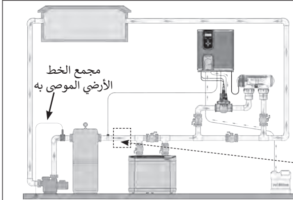
التركيب على الخط
