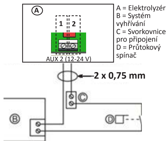
Zapojení systému vyhřívání bez dálkového řízení zapnutí/vypnutí
