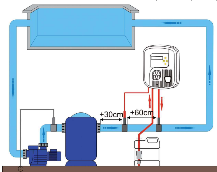
Esquema de instalação Chlor Expert:
