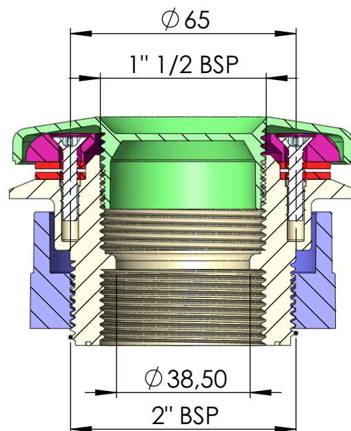
SECCIÓN A-A
