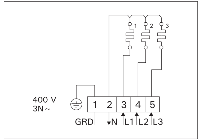
Obrázek 10. Zapojení topného tělesa BX-E
