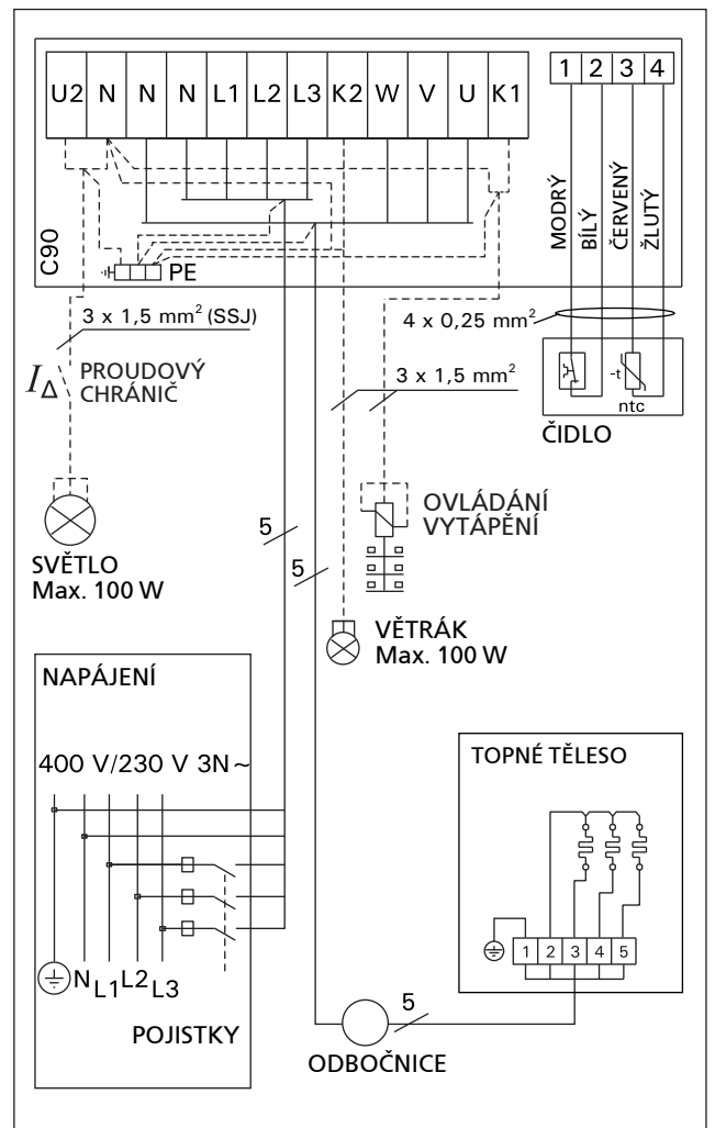
Obrázek 11b. Připojení řídicí jednotky C90 a topidla BX-E k třífázovému napájení
