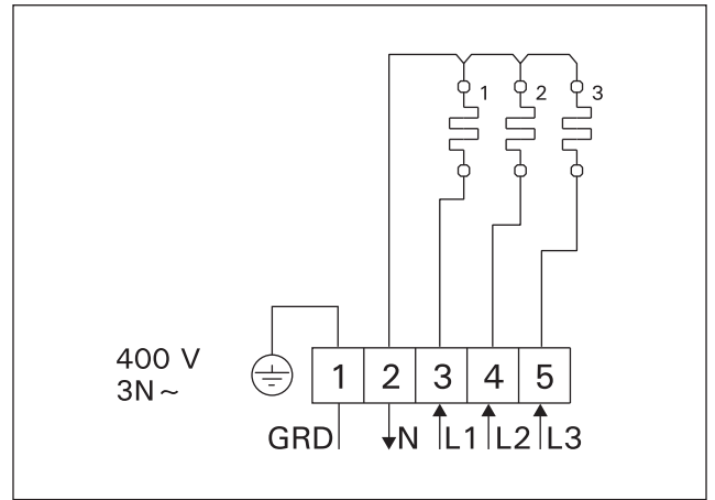
Рисунок 10. Электромонтаж каменки BX-E Joonis 10. BX-E-kerise elektrühendus
