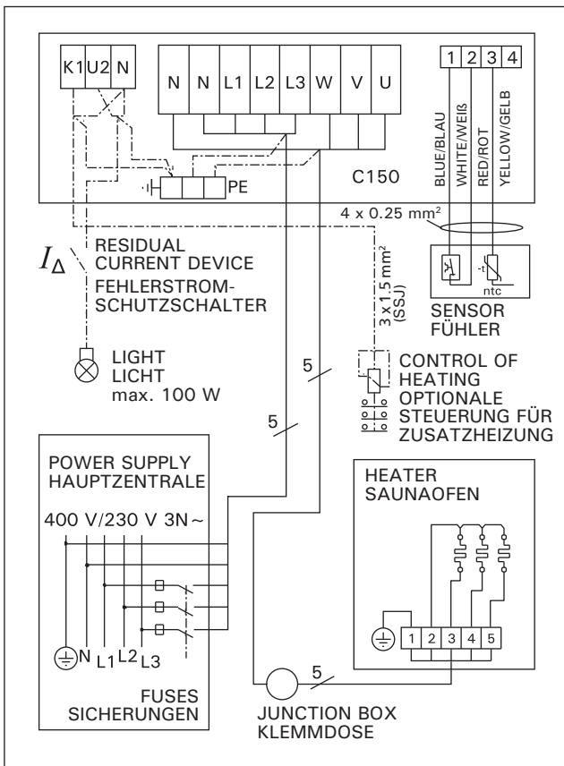
Figure 11a. 3-phase electrical connections of control unit C150 and BX-E-heater Abbildung 11a. 3-phasiger Elektroanschlüsse des Steuergerät C150 und des Saunaofens BX-E
