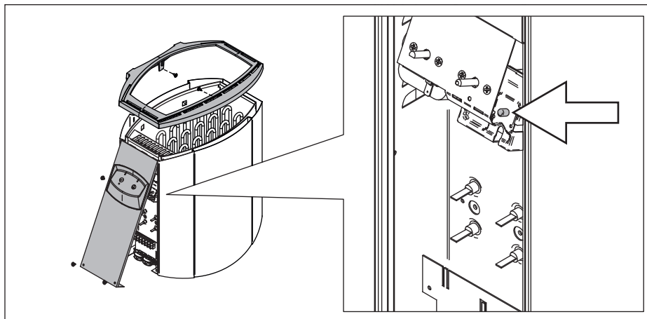
Рисунок 8. Кнопка сброса защиты от перегрева
