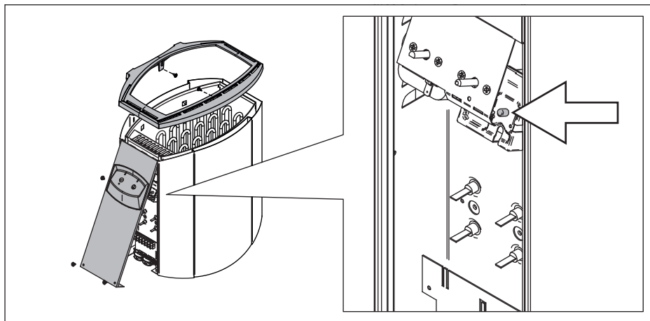
Figure 8. Bouton-poussoir de remise en service de la protection contre la surchauffe Rys. 8. Przycisk resetowania wyłącznika termicznego
