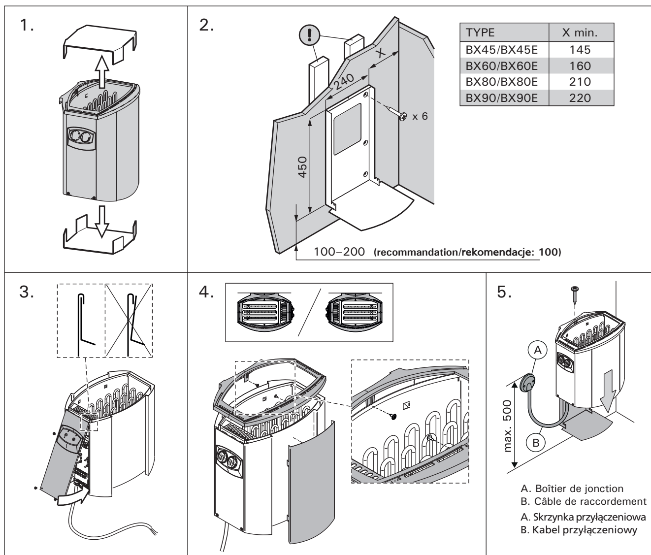
Figure 7. Fixation du poêle au mur (toutes les dimensions sont fournies en millimètres)
