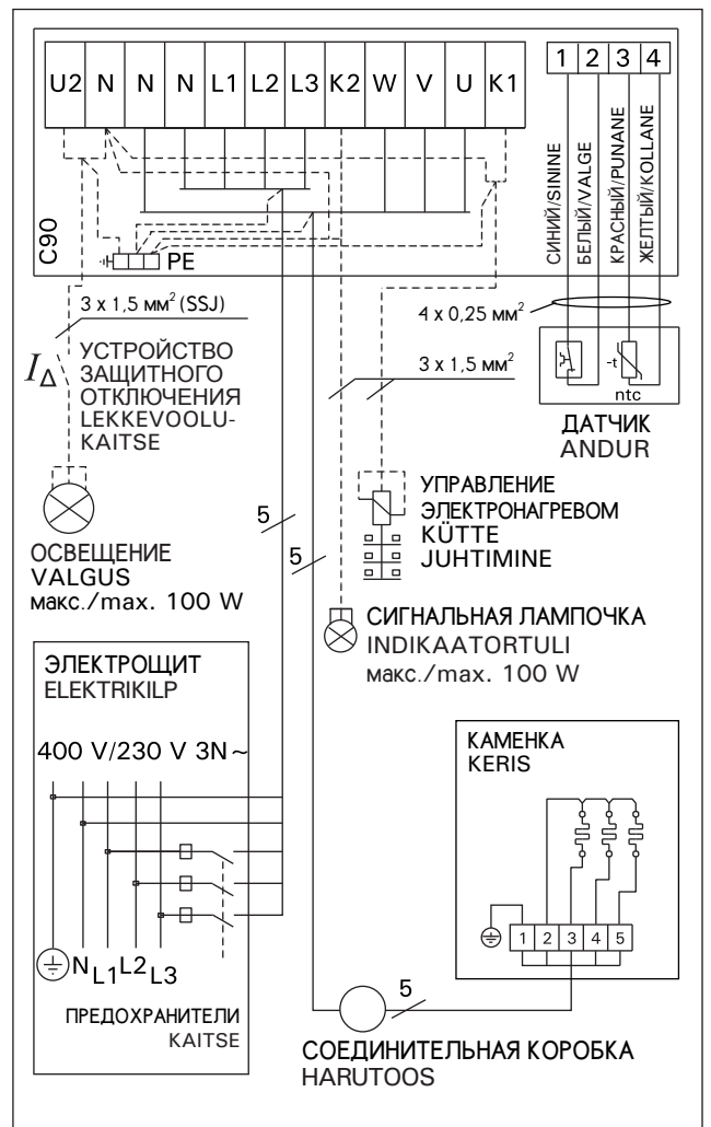
Рисунок 11b. Электромонтаж пульты управления C90 и каменки BX-E (подключение в 3-фазной сети) Joonis 11b. Juhtimiskeskuse C90 ja BX-E-kerise 3-faasilised elektrühendus
