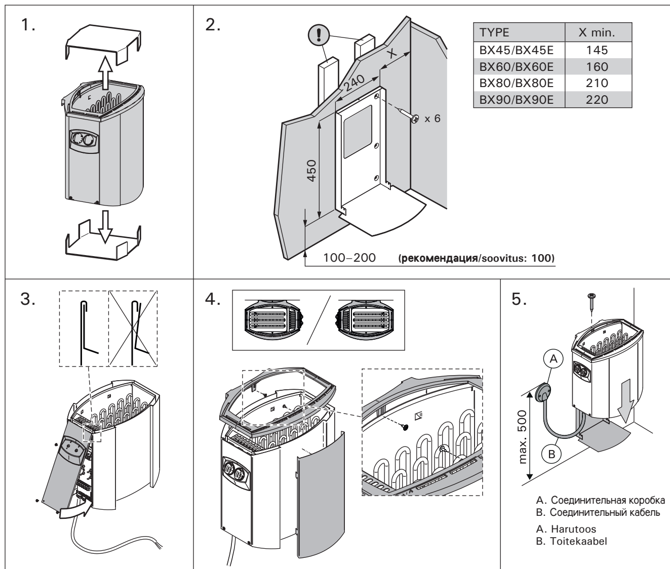
Рисунок 7. Крепление каменки к стене (все размеры приведены в миллиметрах) Joonis 7. Kerise seinalekinnitamine (kõik mõõtmed millimeetrites)
