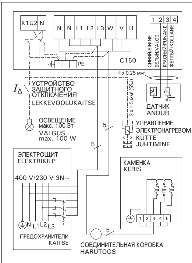
Рисунок 11a. Электромонтаж пульты управления C150 и каменки BX-E (подключение в 3-фазной сети) Joonis 11a. Juhtimiskeskuse C150 ja BX-E-kerise 3-faasilised elektrühendus
