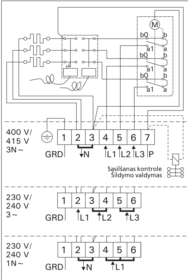
9. zīm. Elektrības pievienošana BX krāsnij 9 pav. BX krosneliņu elektriskā shēma
