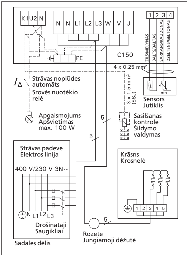
11a. zīm. 3-fāzu elektrības pieslēgums BX-E tipa krāsnij ar C150 distnces vadības pulti 11a pav. Valdymo pultu C150 ir krosnelēs BX-E jungimo j trifazj tīnklā elektriskā shēma
