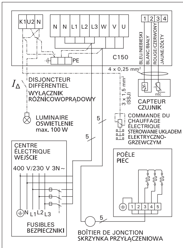
Figure 11a. Centre de contrôle C150 et raccords électriques du poêle BX-E Rys. 11a. Schemat elektryczny pieca typu BX-E i modulu sterujacego C150
