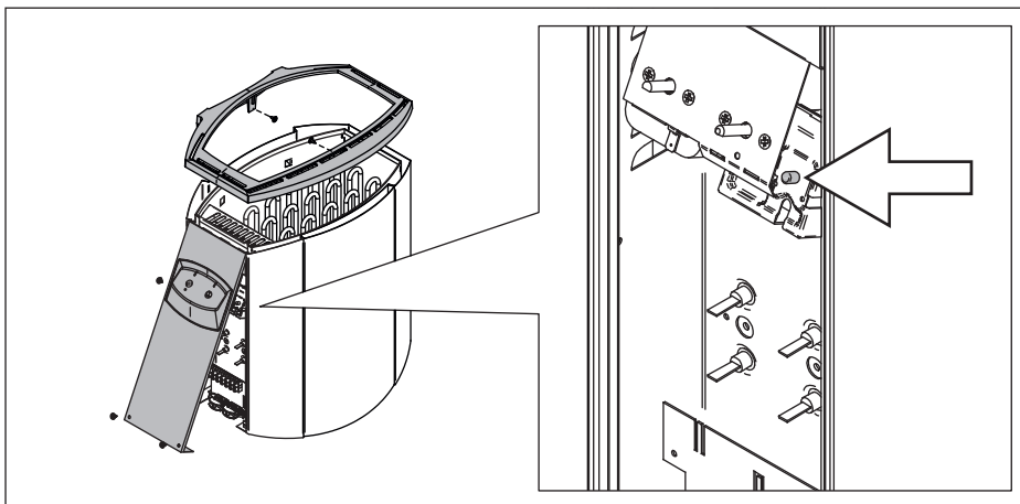
Kuva 8. Ylikuumenemissuojan palautuspainike
