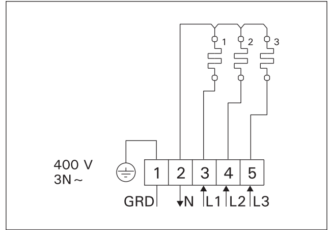
10. zīm. Elektrības pievienošana BX-E krāsnij 10 pav. BX-E krosneliņu elektriskā shēma
