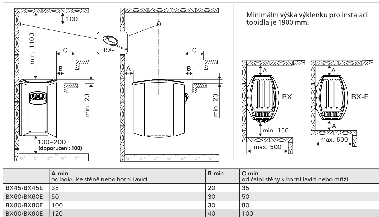
Obrázek 6. Bezpečné vzdálenosti pro topné těleso
