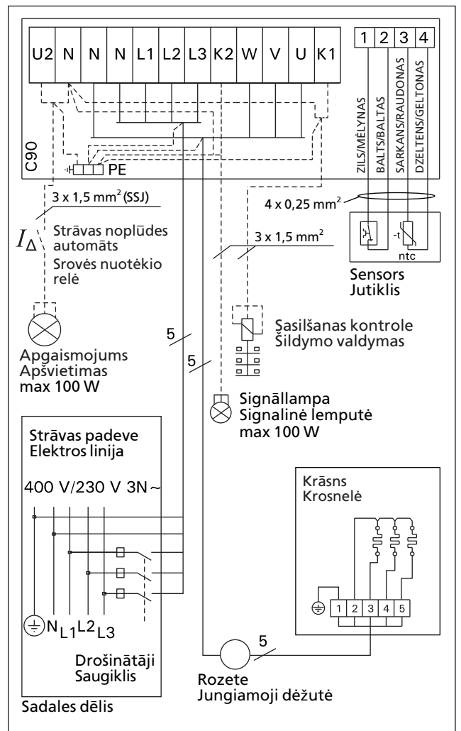
11b. zīm. 3-fāzu elektrības pieslēgums BX-E tipa krāsnij ar C90 distnces vadības pulti 11b pav. Valdymo pultu C90 ir krosnelēs BX-E jungimo j trifazj tīnklā elektriskā shēma
