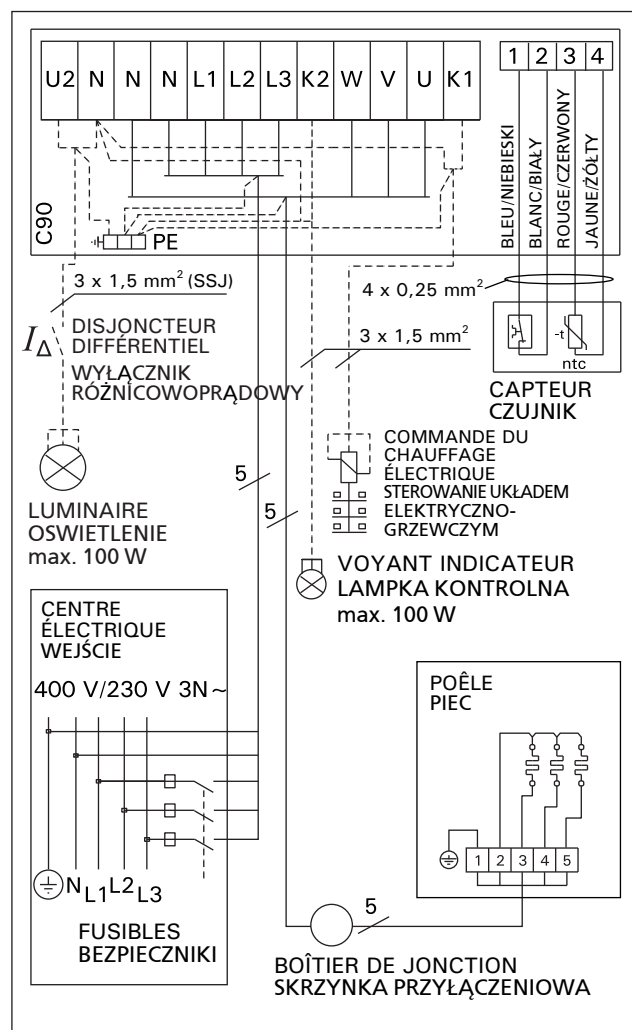
Figure 11b. Centre de contrôle C90 et raccords électriques du poêle BX-E Rys. 11b. Schemat elektryczny pieca typu BX-E i modulu sterujacego C90
