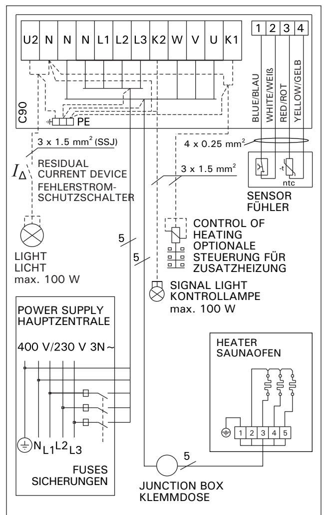
Figure 11b. 3-phase electrical connections of control unit C90 and BX-E-heater Abbildung 11b. 3-phasiger Elektroanschlüsse des Steuergerät C90 und des Saunaofens BX-E
