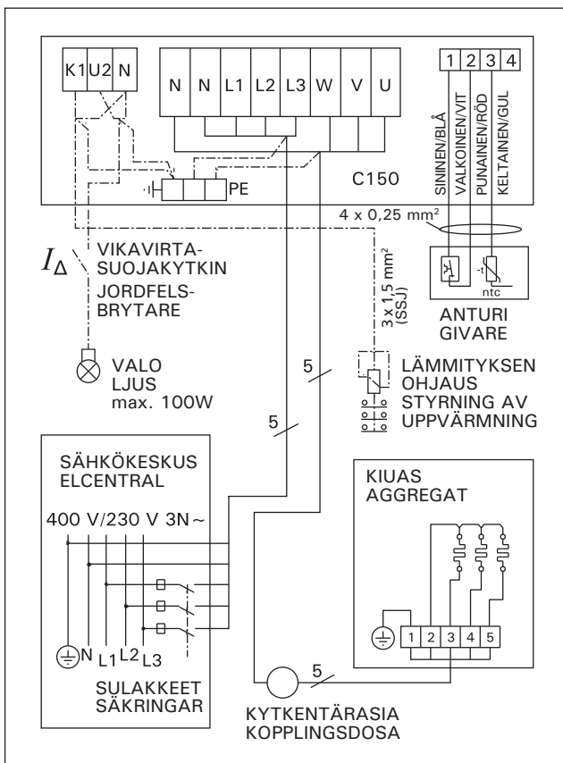
Kuva 11. Ohjauskeskuksen C150 ja BX-E-kiukaan sähkökytkennät Bild 11. Elinstallationer av styrenhet C150 och BX-E-aggregat
