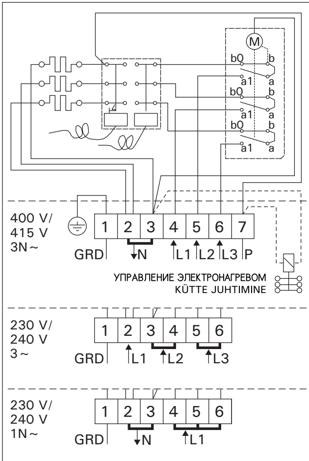
Рисунок 9. Электромонтаж каменки BX Joonis 9. BX-kerise elektrühendus
