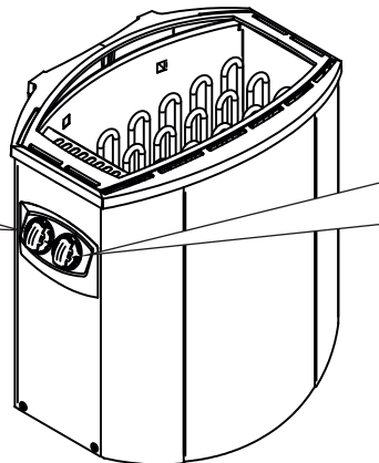
Figure 3. Thermostat switch Abbildung 3. Thermostatschalter
