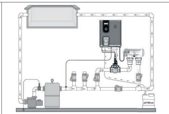
Instalação do eletrolisador + módulo opcional (Exemplo com eXO® (iQ))
