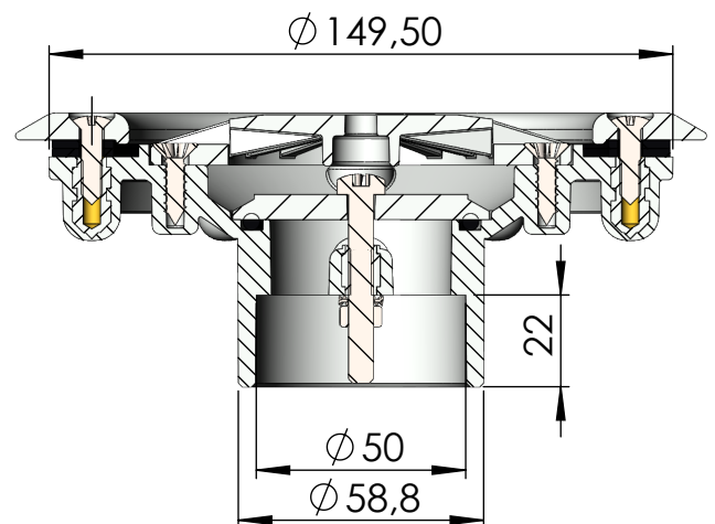
SECCIÓN A-A
