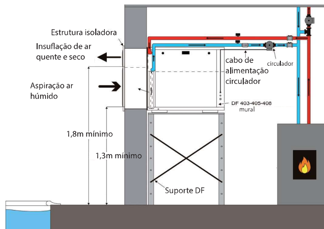
Instalação de uma DF com a opção de bateria de água quente.
