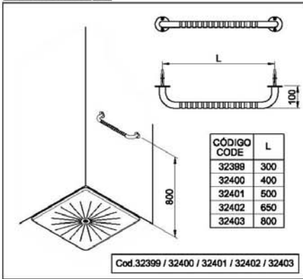
EASYBATH GRAB RAIL POIGNÉE DROITE AGARRADERAS RECTAS
