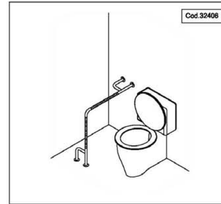
APOYO SUELO FLOOR SUPPORT APPUI DE PLANCHER
