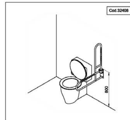
APOYO MURAL ABATIBLE SUPPORT FOR FOLDING WALL L'APPUI POUR PLIER LE MUR
