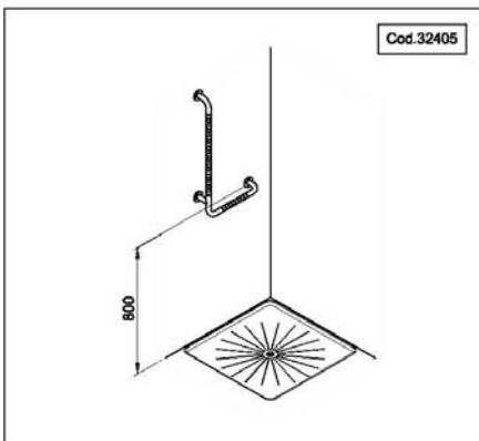
ANGULAR GRAB RAIL POIGNÉE ANGOLAIRE SUJECIÓN ANGULAR VERTICAL
