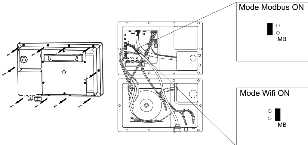
Mode Modbus : Les voyants LED Wifi et Bluetooth clignotent simultanément.
