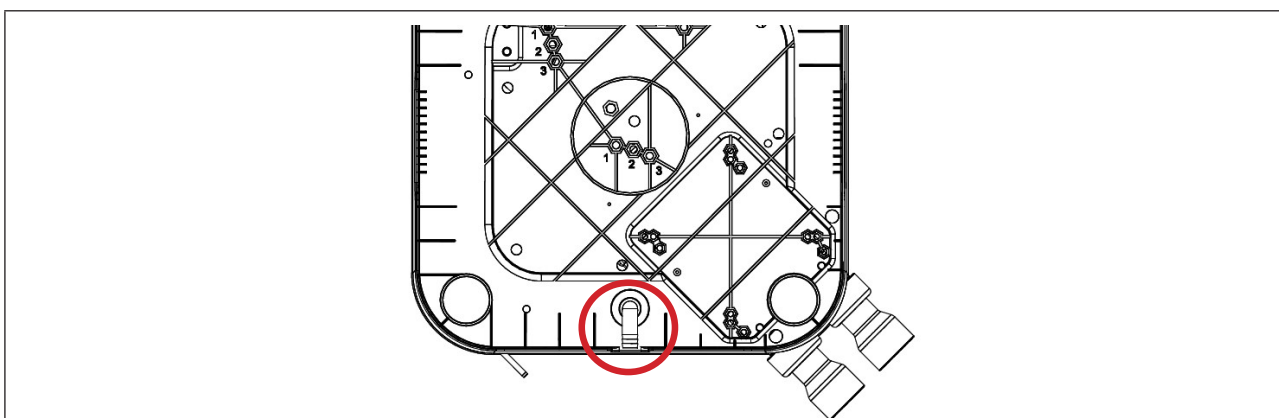
Orientation de l'évacuation des condensats (vue du dessous de l'appareil)
