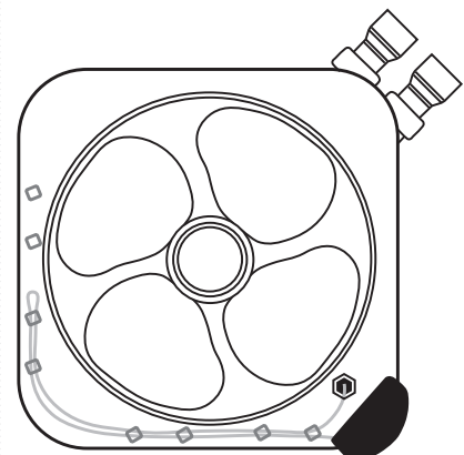
Recorrido del cable al girar la interfaz de usuario hacia la derecha
