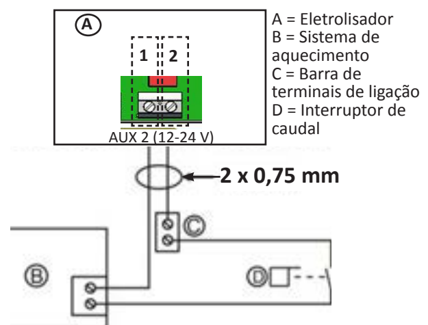
Ligação de um sistema de aquecimento sem controlo "ligar/ desligar" à distância
