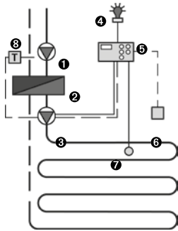
Abb. 90 Schaltschema
