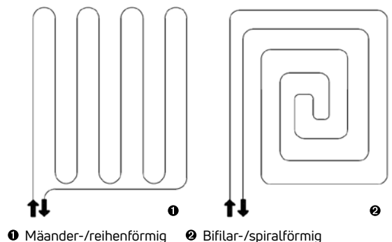
Abb. 136 Verlegeschema
