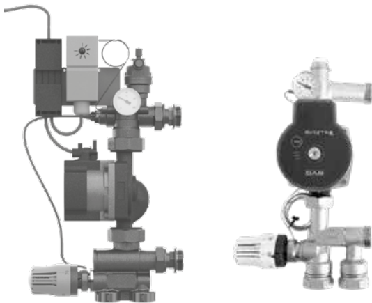
Abb. 113 Festwertregelsets TempCo fix eco 3 (links) und Objekt line
