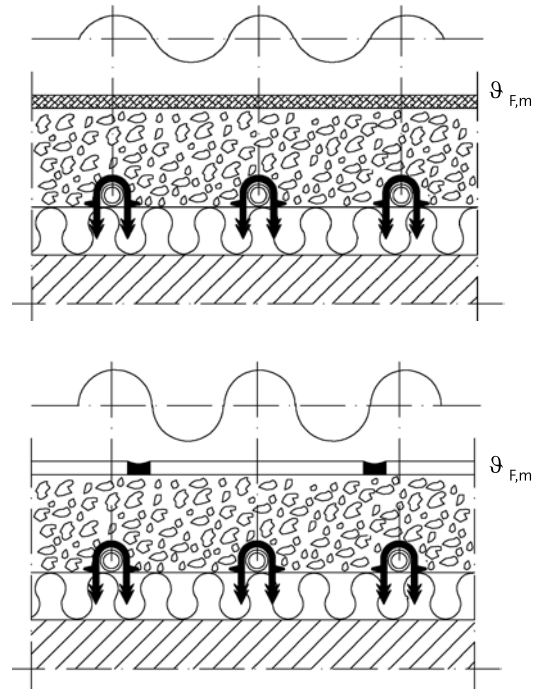
Abb. 133 Temperaturen in der Fußbodenheizung
