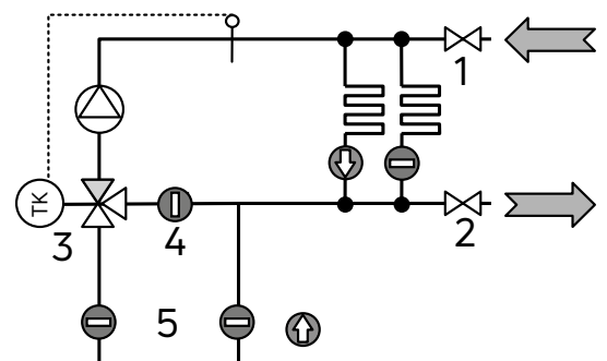
Abb. 116 Füllen und Spülen der einzelnen Heizkreise
