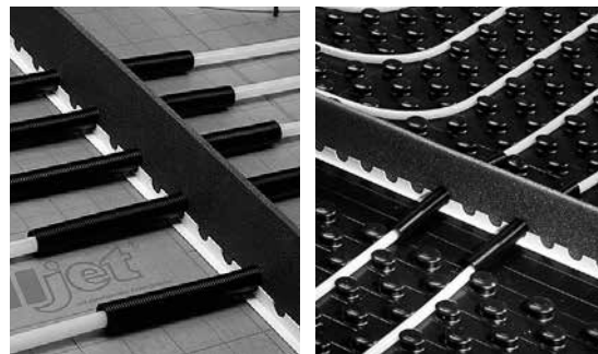
Abb. 130 Dehnfugenprofil rolljet (links) sowie Dehnungsfugenprofil und Übergangselement noppjet uni (rechts)
