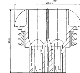
Schnitt A-B
