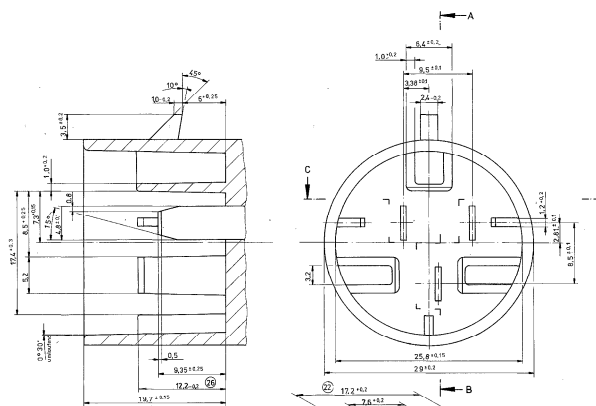
Schnitt A-B
