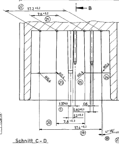
Schnitt C - D
