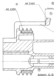
Schnitt C-D
