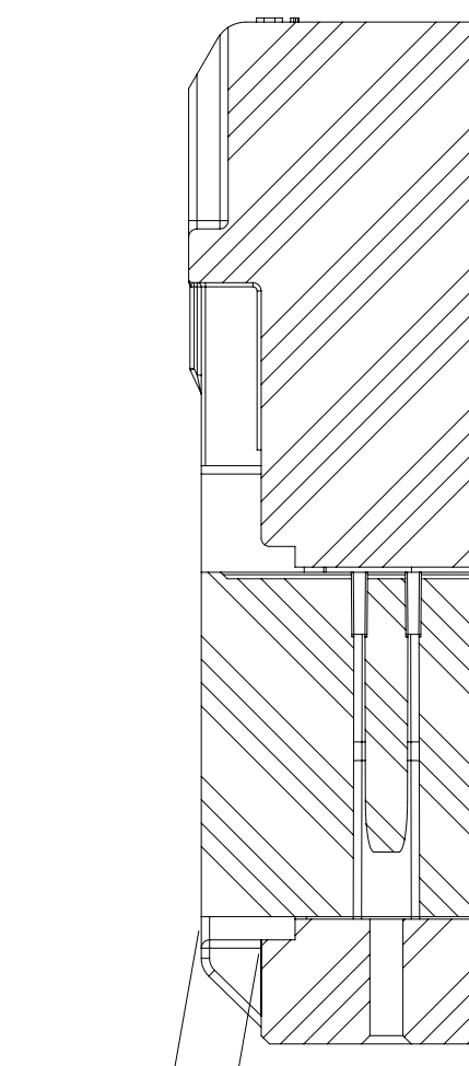
SECTION A-A
